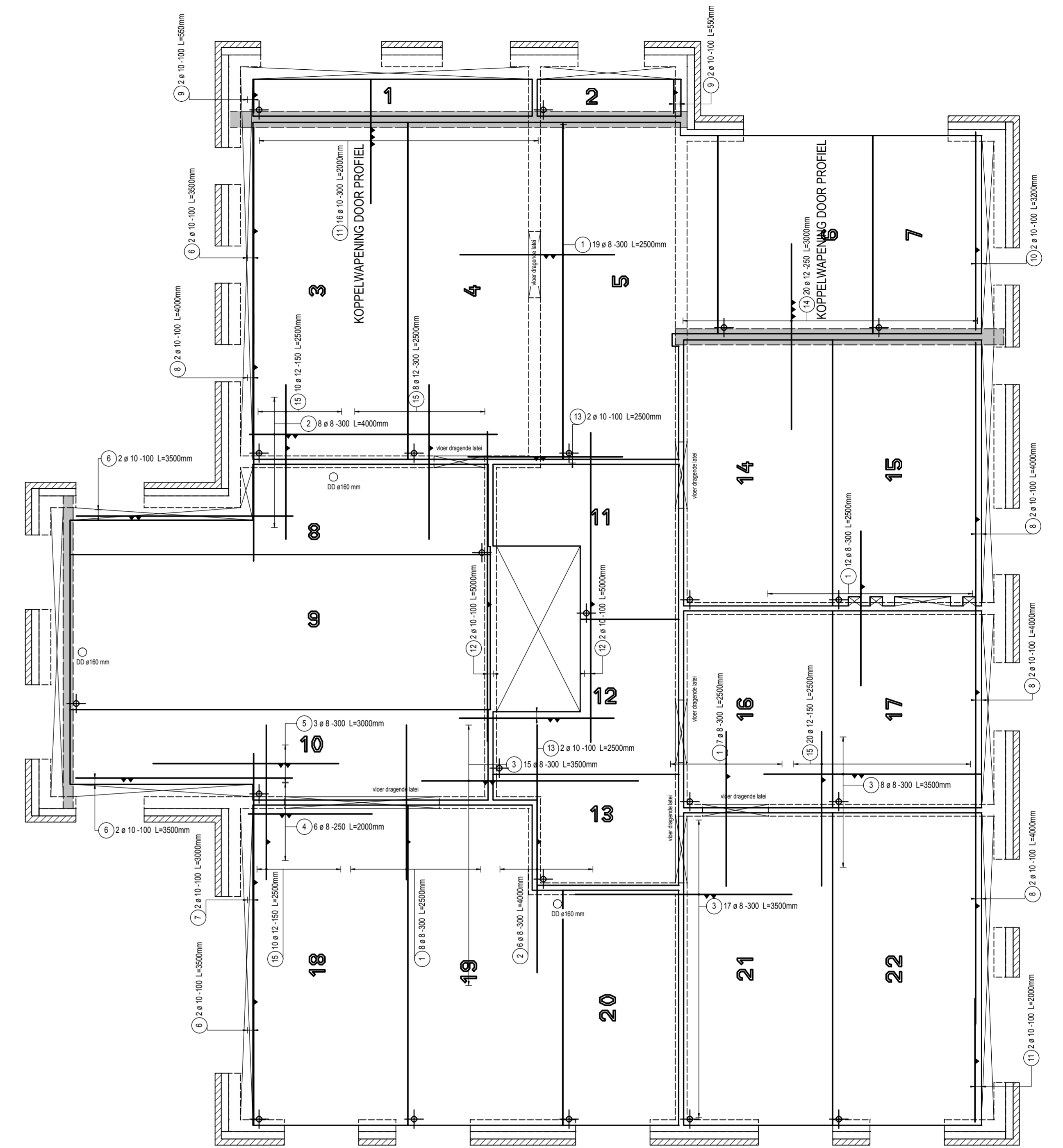
BOVENWAPENING BIJLEGSTAVEN DEKKING 15MM
