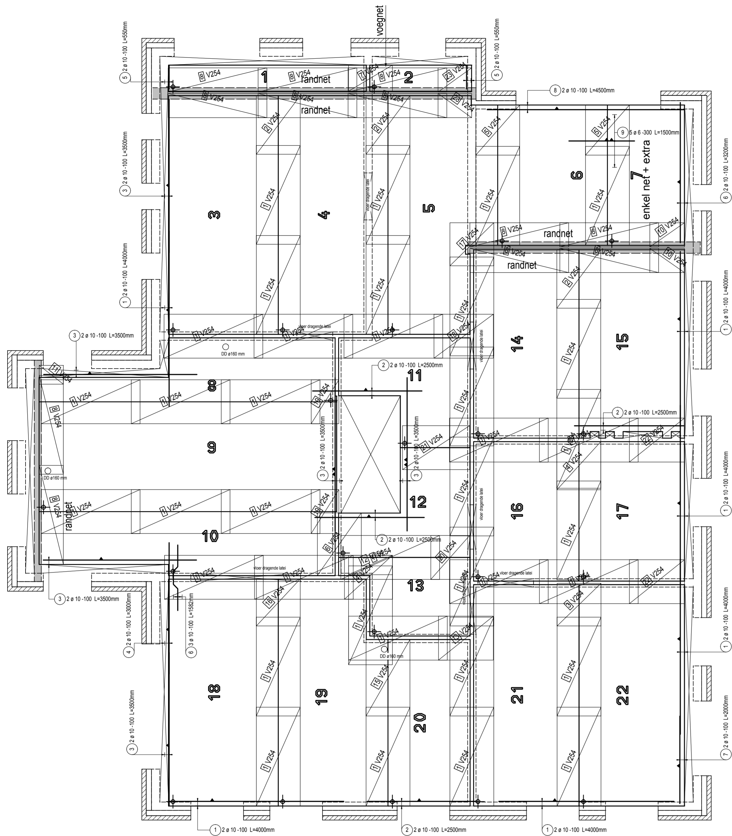
VOEGWAPENING OP DE SCHIL AANBRENGEN
